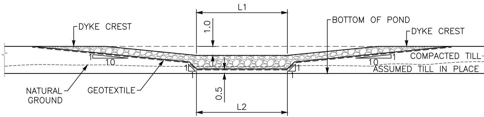
SECTION D-D
