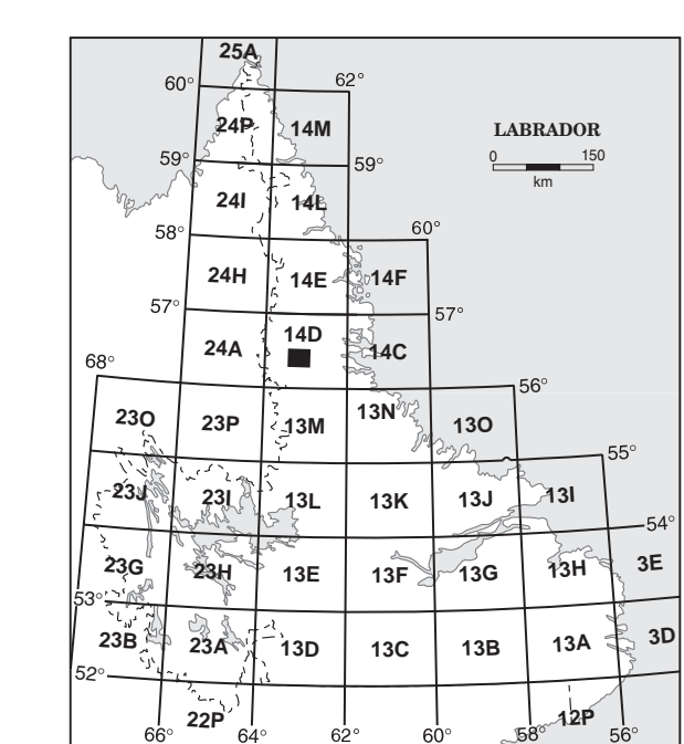
INDEX MAP
